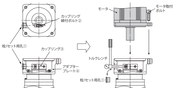
図 5-1 組付図
