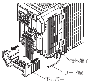
図 9 リード線と接地端子の接続
