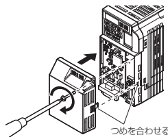
図 14 オプションカバーの取付け
