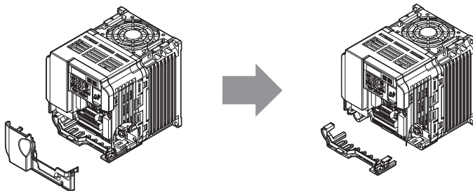
図 11 端子カバー付モデルの取付け方法
