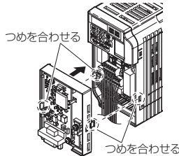
図 12 オプションユニットの取り付け
