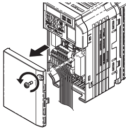
図 8 フロントカバーの取り外し
