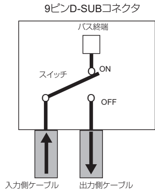
図 6 PROFIBUS コネクタと終端抵抗
