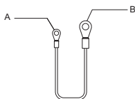
図 10 リード線の詳細
