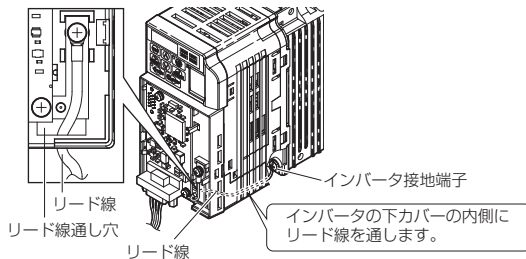
図 13 リード線の接続
