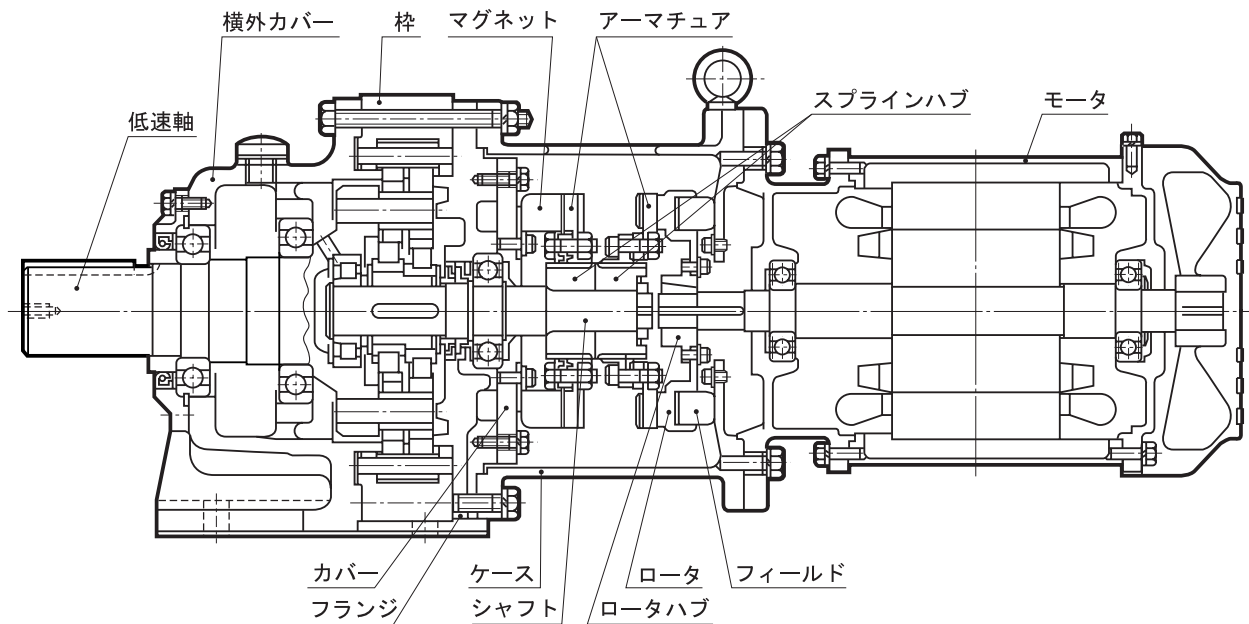
図 10-2 CHHCM 形(例: CHHCM8-6175-EP)
