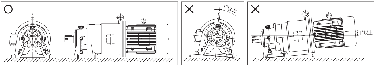
図 4-1 据付角度(例：脚付)
