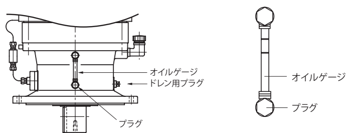
図 8-3 排油
