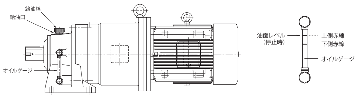
図 8-1 横形
