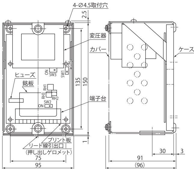
外形寸法図
