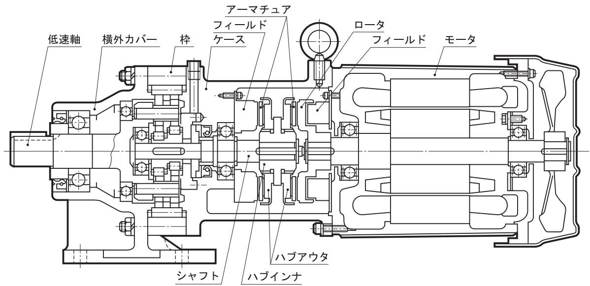
図 10-1 CHHCM 形(例: CHHCM1-6105-EP)
