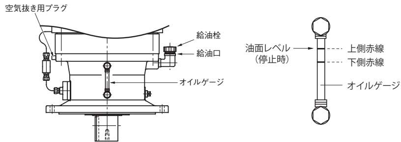
図 8-2 立形
