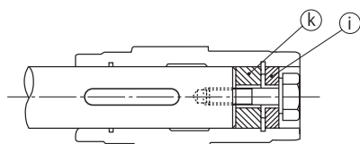
図F14 固定方法
