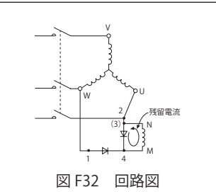
■普通制動回路
