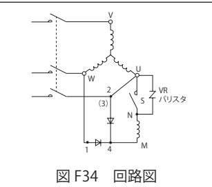
■急制動回路
