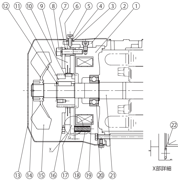
図 F40 FB-1HE、FB-2E（屋内形）
