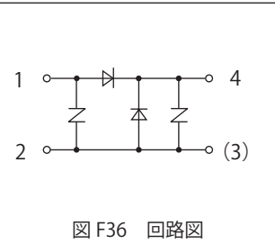
■整流器内部回路図（参考）
