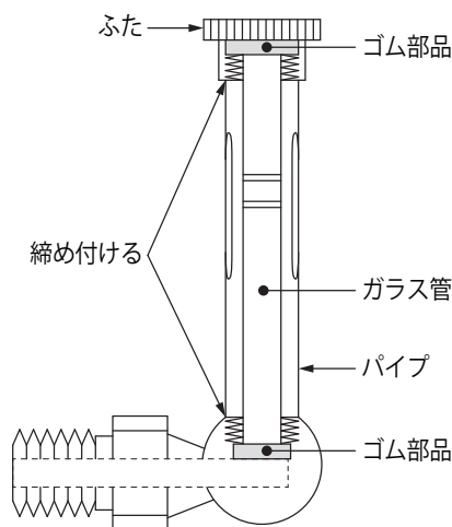
図 8-4 L 形オイルゲージ
