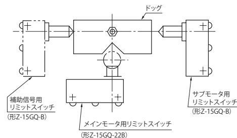
図 11-1 リミットスイッチ
