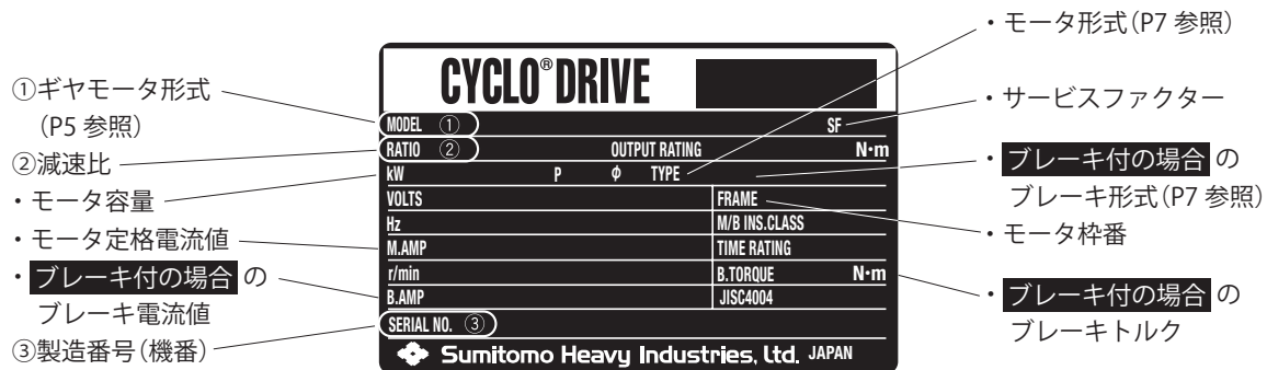
図 1-1 ギヤモータの銘板 (タイプ1)
