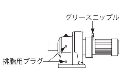
図 8-6 給排脂口の位置 (例：横形・ギヤモータ・2 段形)
