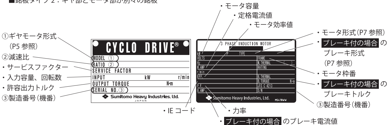
図 1-2 ギヤモータの銘板 (タイプ2)
