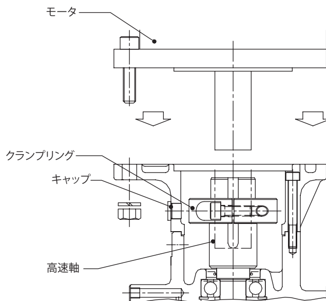
図 4-2 組付図
