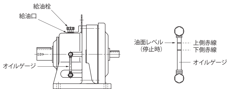
図 8-2 横形
