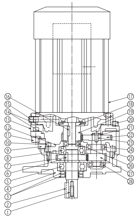
図 10-16 CVVM 形 (6000SK シリーズ・SL シリーズ立形・ギヤモータ) (例：枠番 6075SK)
