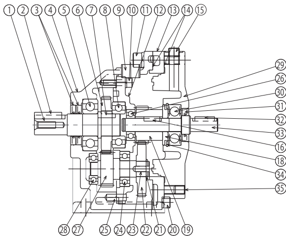
図 10-17 CHH 形 (6000SK シリーズ・SL シリーズ横形・レデューサ) (例：枠番 6075SK)
