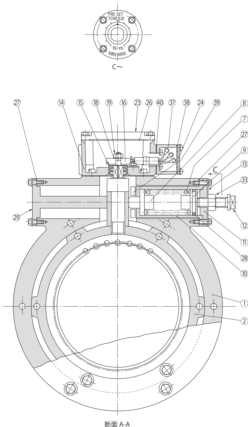
図 15-2 CHHM 形（横形・ギヤモータ）、3 段形
