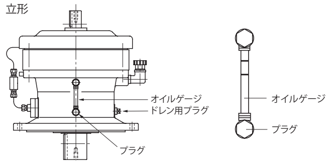
図 8-5 排油
