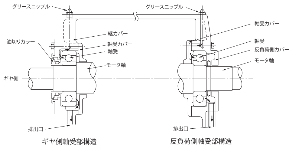
図 8-9 開放形軸受部構造
