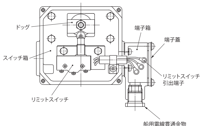
図 11-2 端子箱・スイッチ箱
