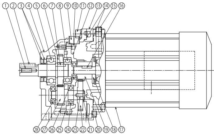
図 10-15 CHHM 形 (6000SK シリーズ・SL シリーズ横形・ギヤモータ) (例：枠番 6075SK)
