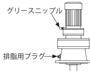
図 8-7 給排脂口の位置 (例：立形・ギヤモータ・2 段形)
