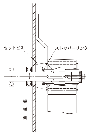
図 14. セットビスとストッパリングによる固定 (被動軸段なし)
