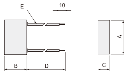
■外形寸法図
