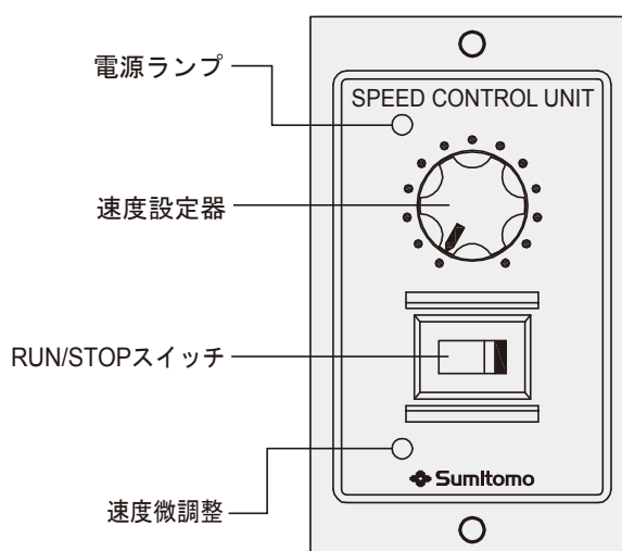
図 1. ユニットタイプスピードコントローラの正面図
