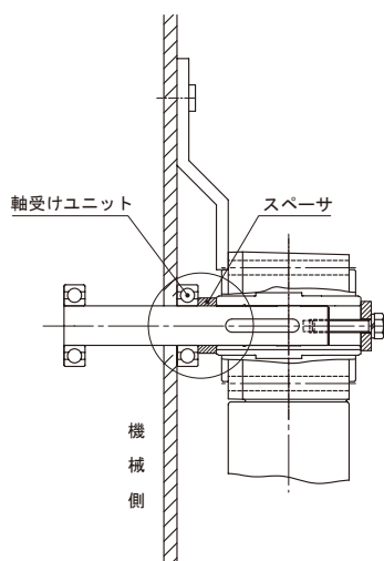
図 13. スペーサによる固定 (被動軸段なし)
