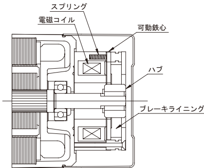
図 1. 電磁ブレーキ付モータの構造
