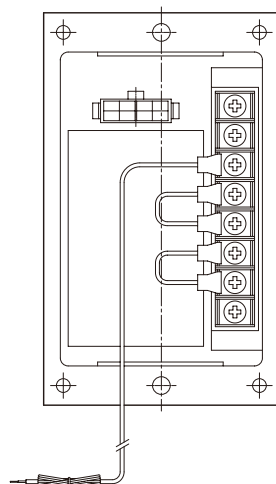
スイッチボックス（1φ）背面図
