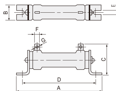
■外形寸法図
