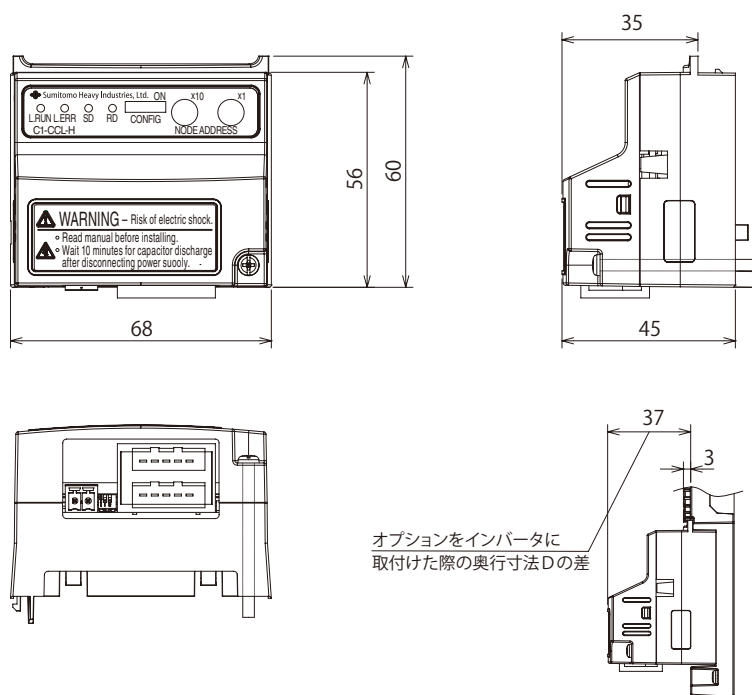
取付図
