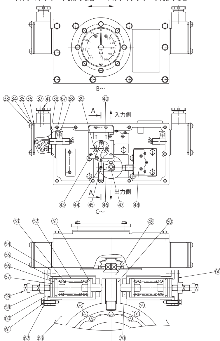
図 15-3 トルクインジケータ
