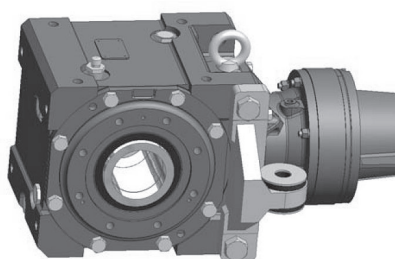
アタッチメントタイプトルクアーム(オプション)
