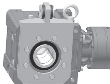
バンジョータイプトルクアーム(オプション)
