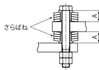
図 5-12 さらばね
